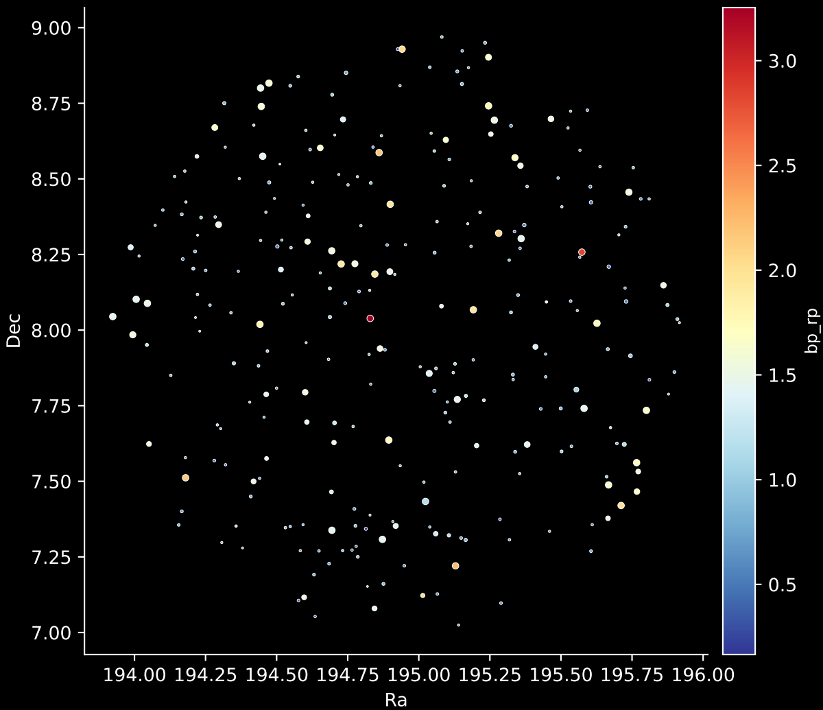
GALAH DR4 Field: [9470] Stars: 280
