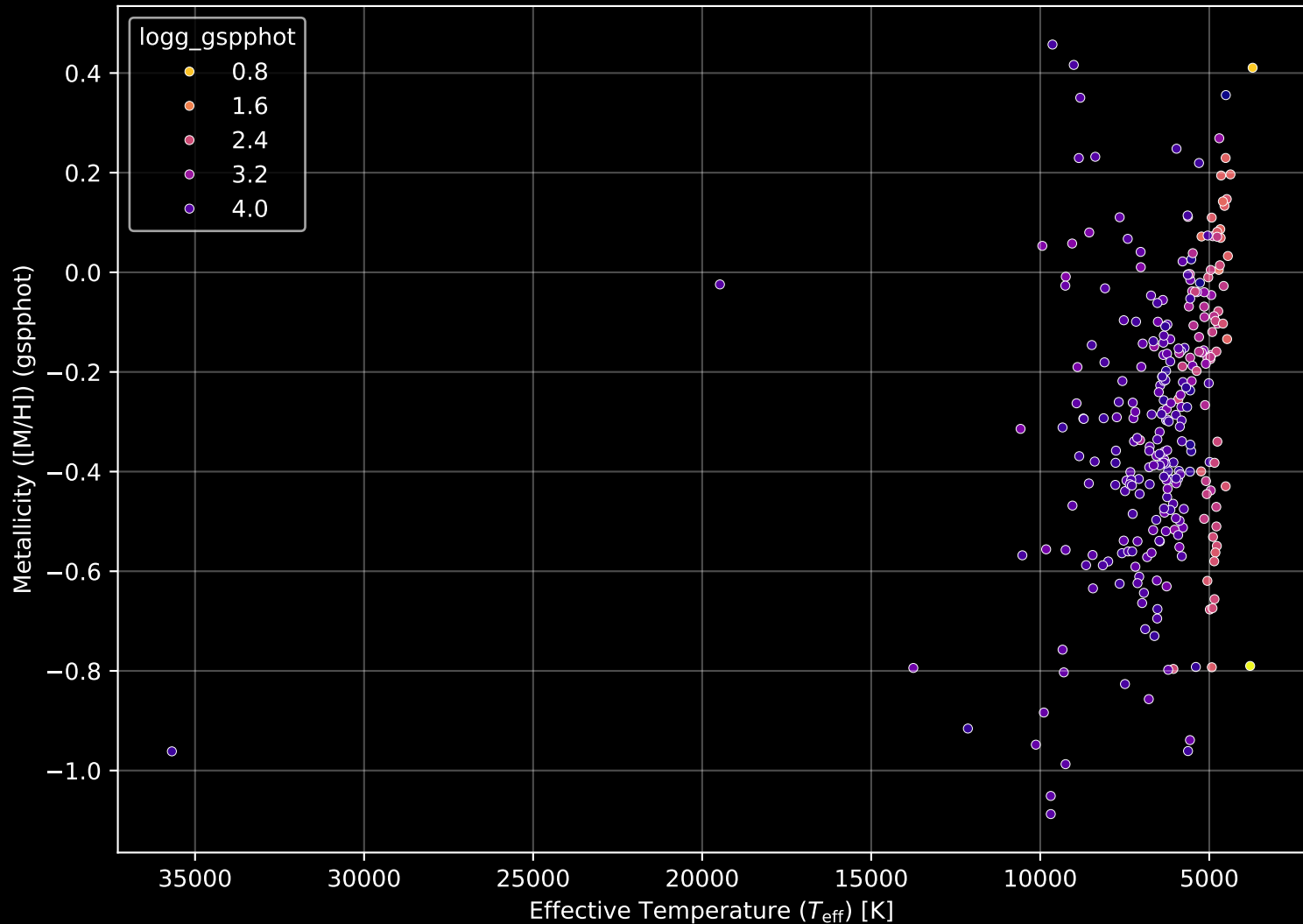
GALAH DR4 Field: [9470] Stellar Population Parameters (n= 280)
